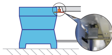
SGブリッジの浮き上がり防止機能を必ず使用してください。
