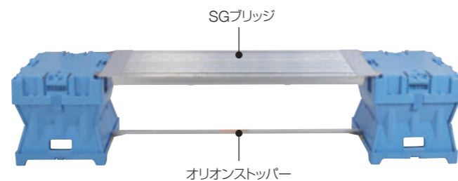
オリオンストッパー<下部連結棒> 長さ:1510mm 重量:600g
